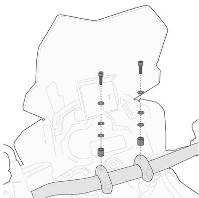
04SKITK Kit de fixation spécifique pour Smart Bar KS900A
